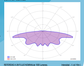
CURVAS POLARES
